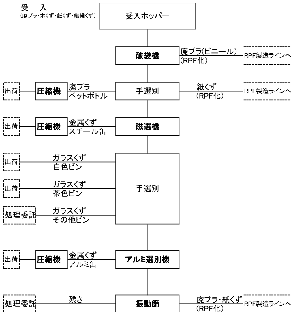
缶・ビン・ペットボトル選別・圧縮ライン 処理工程図
